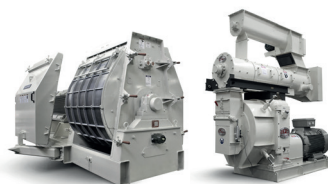
PELLETSPRESSAR & HAMMARKVARNAR
